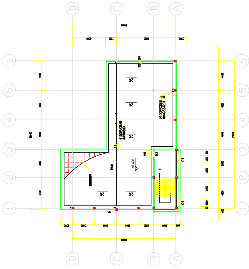
天面平面圖
